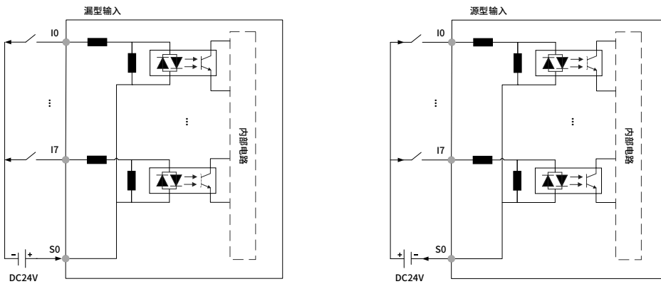
图 8 本地输入内部电路图
