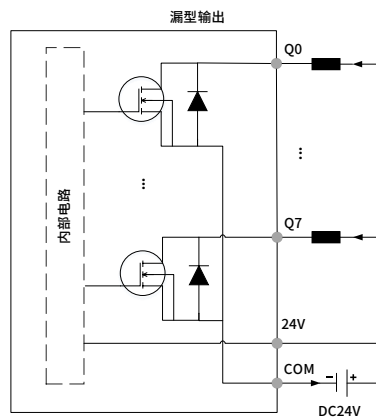
图 9 本地输出内部电路图
