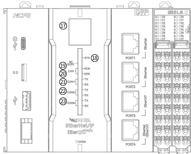
图 4 HCQ9P 状态指示灯说明图
