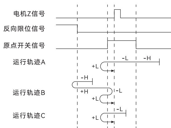
图 22. 模式 13 原点回零运行轨迹示意图
