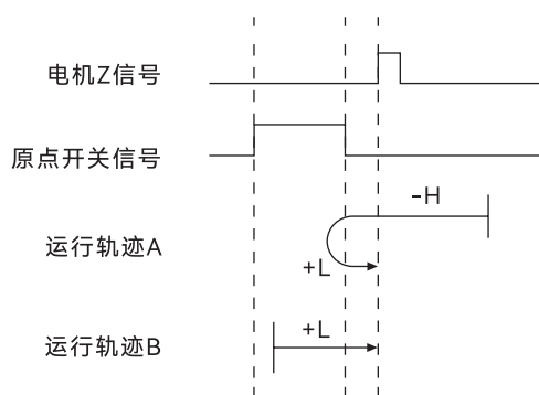
图 14. 模式 5 原点回零运行轨迹示意图
