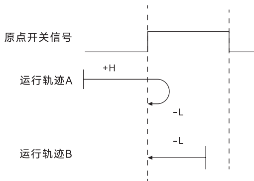
图 26. 模式 19 原点回零运行轨迹示意图
