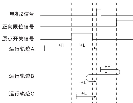
图 19. 模式 10 原点回零运行轨迹示意图
