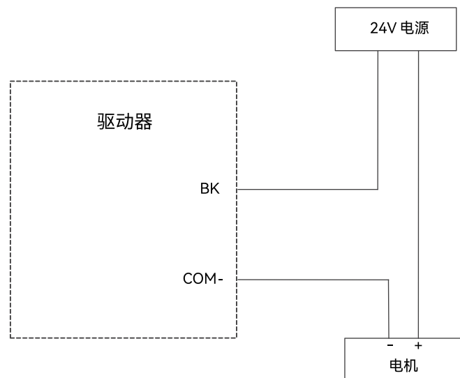
图 3. AMD520B-2D715、AMD520B-2D725、AMD520B-2D760、AMD520B-2D784 电机刹车接线图
