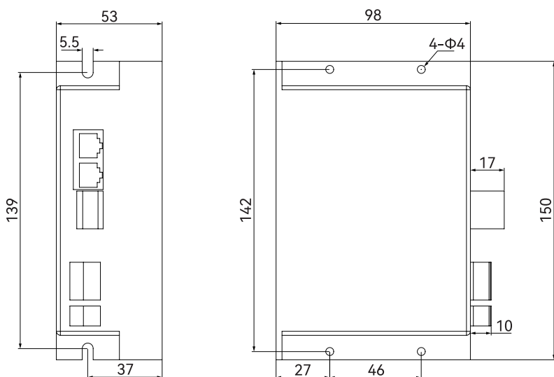
图 2. SIZE B 外形尺寸图 (单位: mm)
