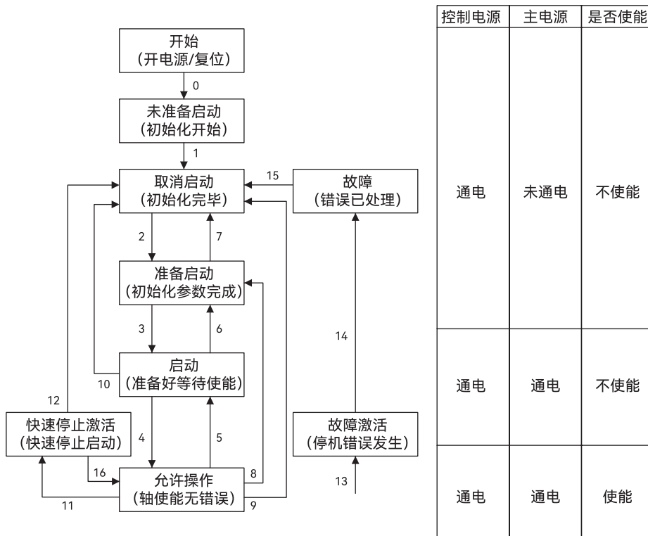
图 5. CIA402 状态机
