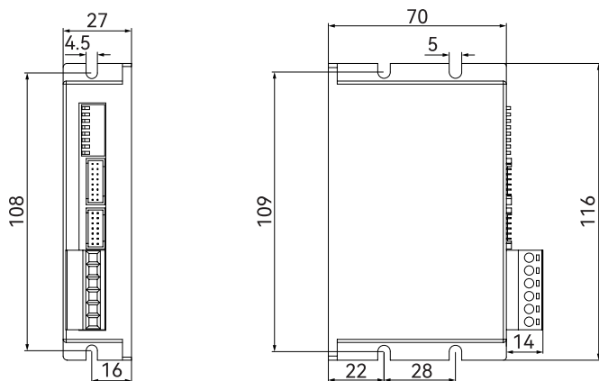
图 1. SIZE A 外形尺寸图 (单位: mm)
