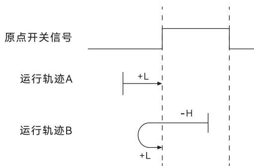
图 27. 模式 20 原点回零运行轨迹示意图
