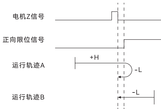
图 11. 模式 2 原点回零运行轨迹示意图
