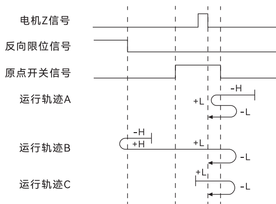
图 21. 模式 12 原点回零运行轨迹示意图
