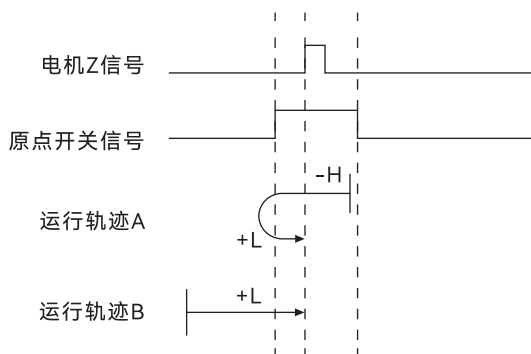
图 13. 模式 4 原点回零运行轨迹示意图
