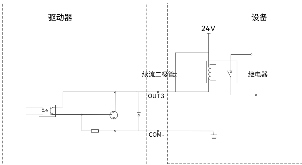
图 3. AMD520B-2D715、AMD520B-2D725、AMD520B-2D760、AMD520B-2D784 电机刹车接线图
