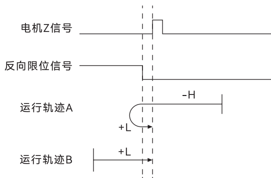
图 10. 模式 1 原点回零运行轨迹示意图
