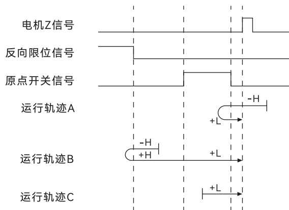
图 20. 模式 11 原点回零运行轨迹示意图
