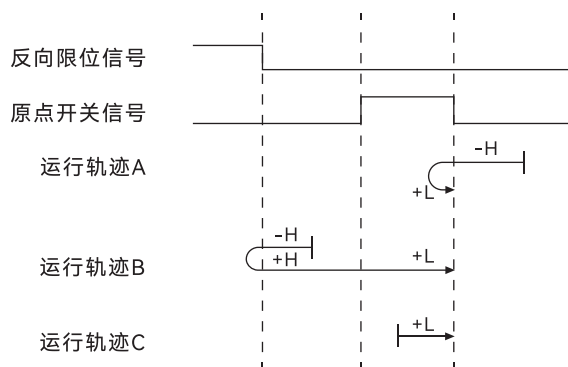
图 34. 模式 27 原点回零运行轨迹示意图
