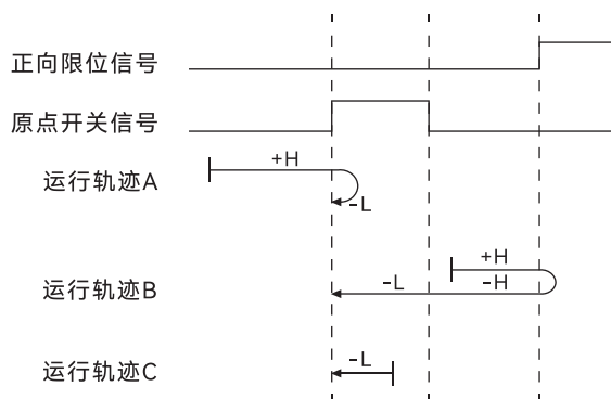
图 30. 模式 23 原点回零运行轨迹示意图
