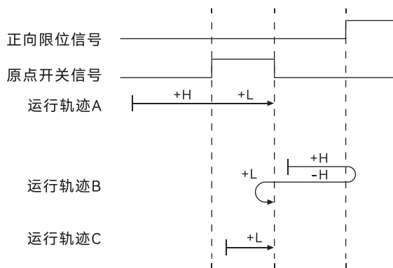
图 33. 模式 26 原点回零运行轨迹示意图
