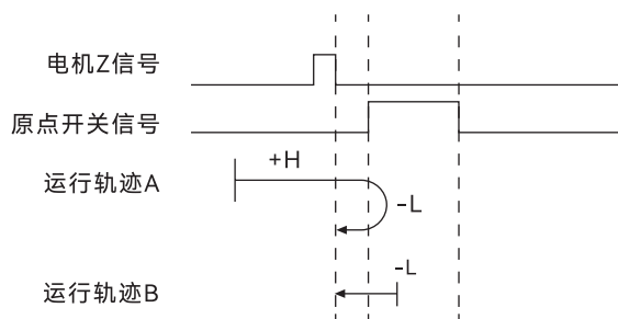
图 12. 模式 3 原点回零运行轨迹示意图
