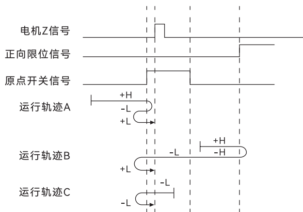
图 17. 模式 8 原点回零运行轨迹示意图
