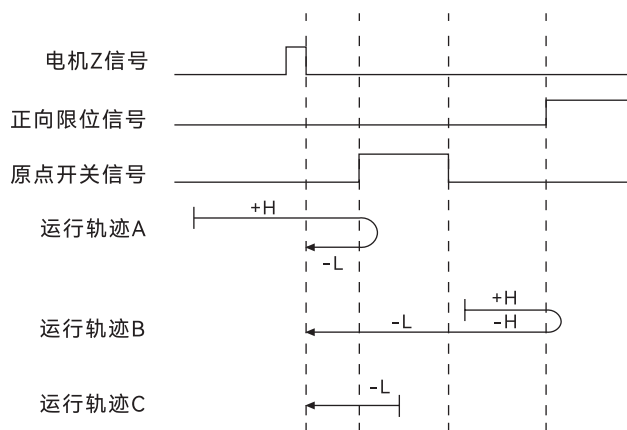
图 16. 模式 7 原点回零运行轨迹示意图
