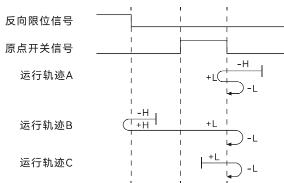
图 35. 模式 28 原点回零运行轨迹示意图
