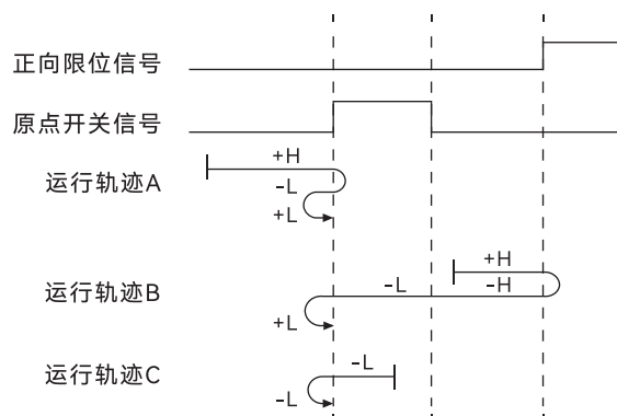
图 31. 模式 24 原点回零运行轨迹示意图
