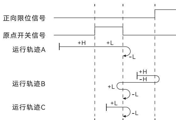
图 32. 模式 25 原点回零运行轨迹示意图
