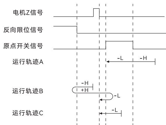
图 23. 模式 14 原点回零运行轨迹示意图
