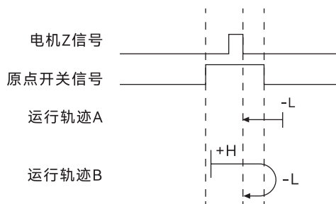
图 15. 模式 6 原点回零运行轨迹示意图
