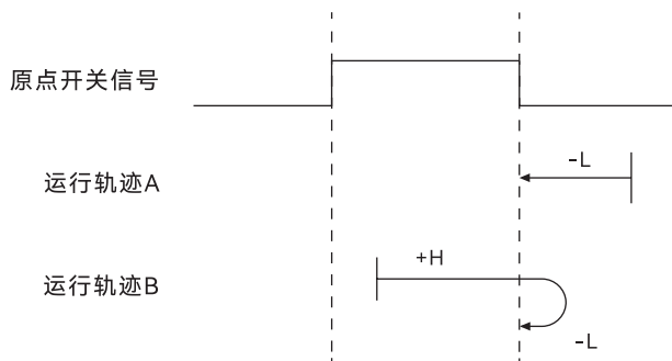
图 29. 模式 22 原点回零运行轨迹示意图
