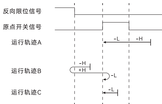
图 37. 模式 30 原点回零运行轨迹示意图
