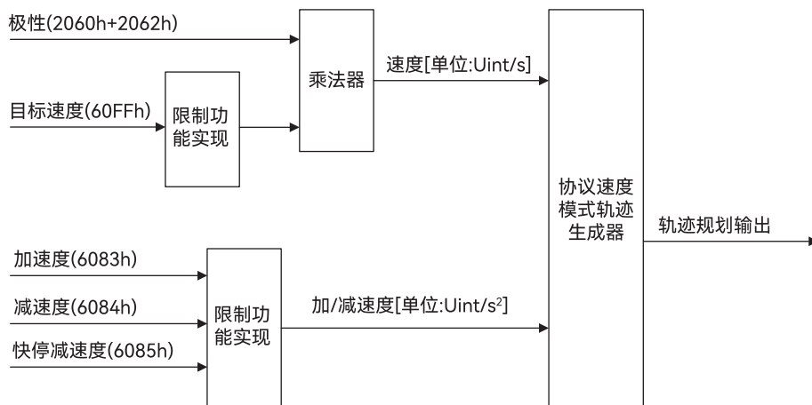
图 9. PV 模式的轨迹生成
