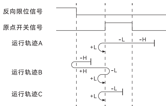
图 36. 模式 29 原点回零运行轨迹示意图
