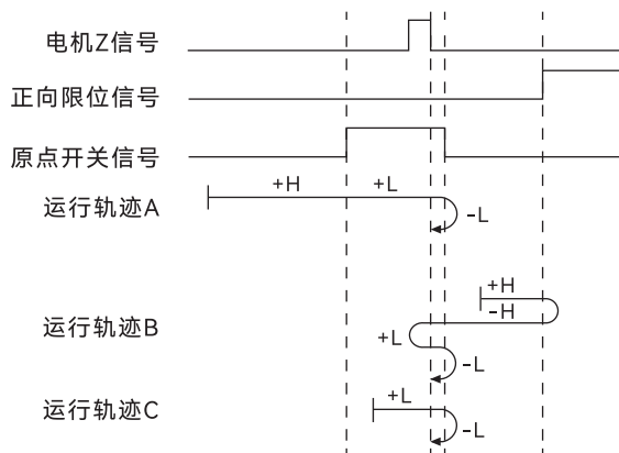
图 18. 模式 9 原点回零运行轨迹示意图
