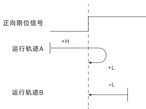
图 25. 模式 18 原点回零运行轨迹示意图
