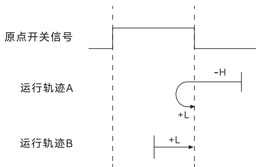
图 28. 模式 21 原点回零运行轨迹示意图
