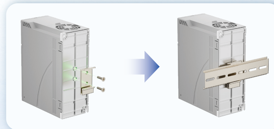
导轨安装*
