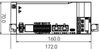
仰视图
