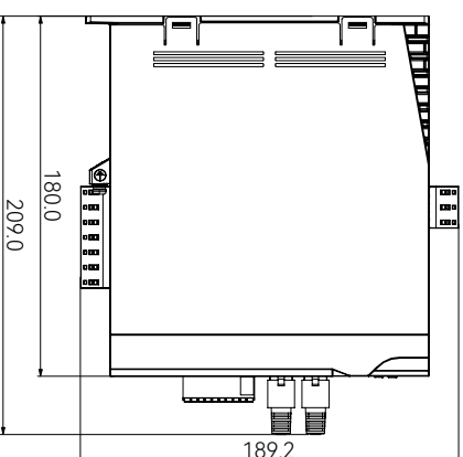
左视图
