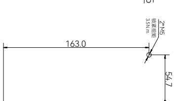
安装孔位图
