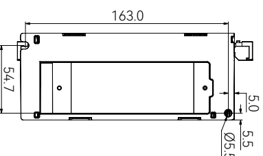
后视图
