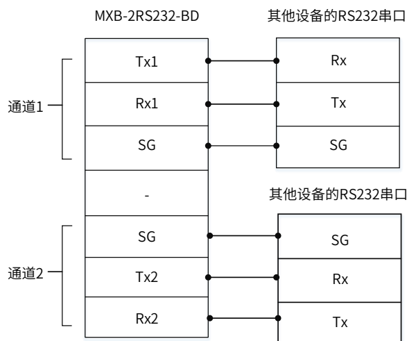
图 6 HCMXB-2RS232-BD 通信连接图
