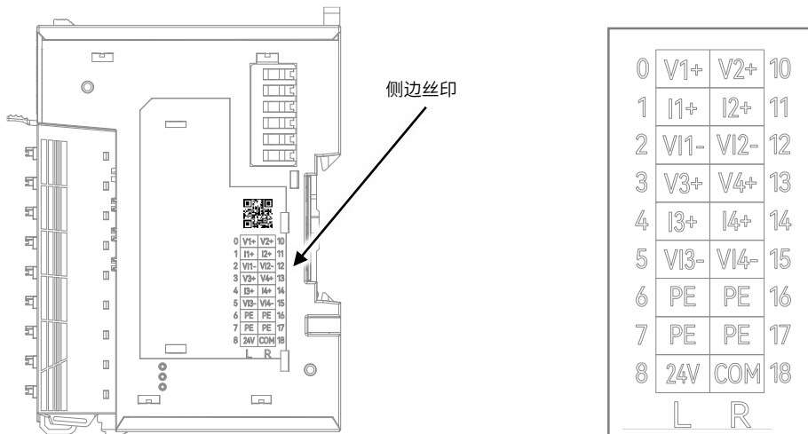
图 4 HCMX-AD04-D 模块侧边丝印
