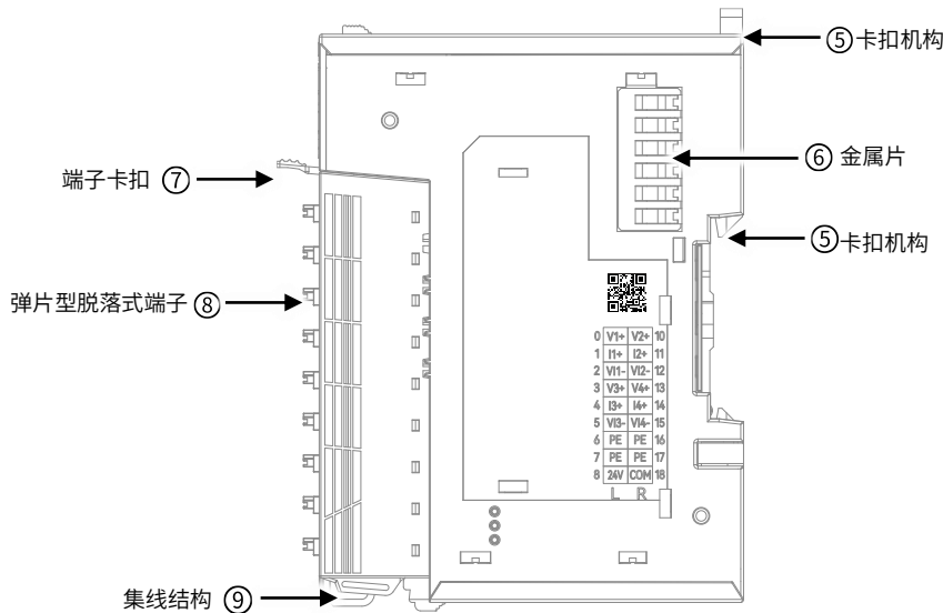
图3 HCMX-AD04-D 模块右视图
