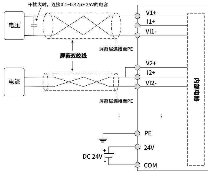
图 6 HCMX-AD04-D 模块内部接线图
