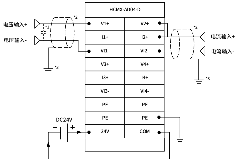
图 7 HCMX-AD04-D 模块端子接线图
