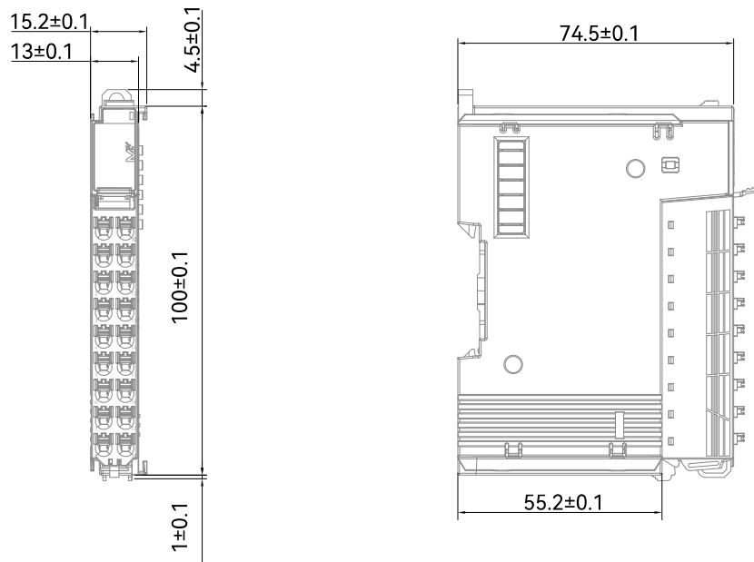
图5 HCMX-AD04-D 模块尺寸图
