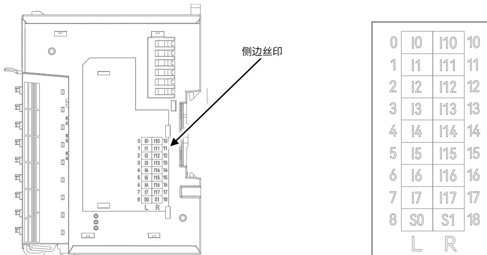
图 4 HCMX-ID16-D 模块侧边丝印
