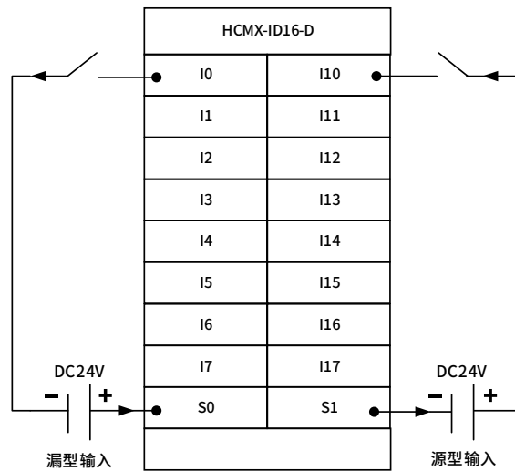
图 7 HCMX-ID16-D 模块端子接线图
