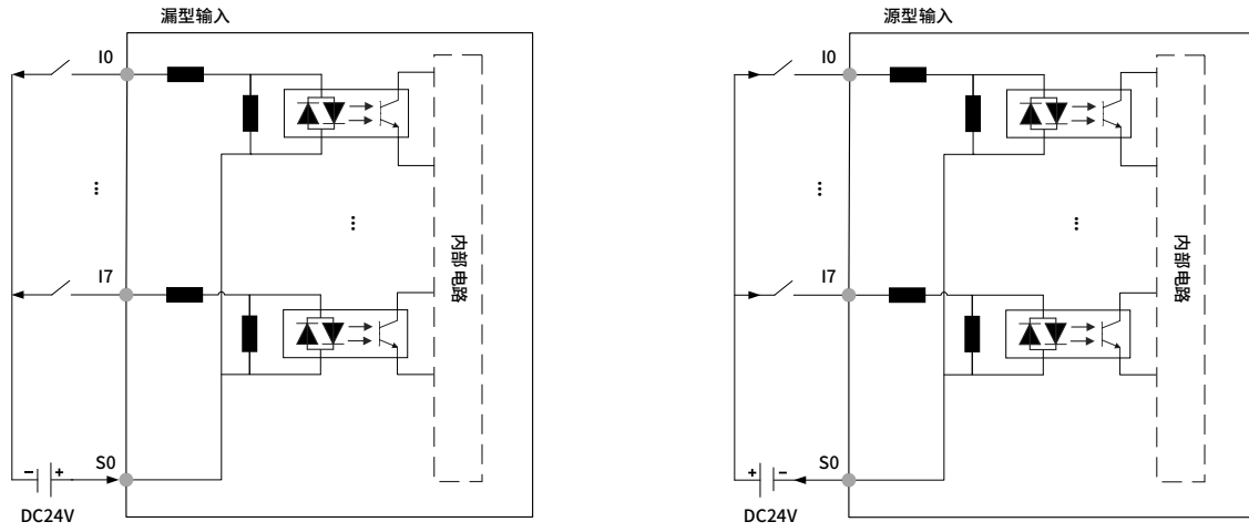
图 6 HCMX-ID16-D 模块内部接线图
