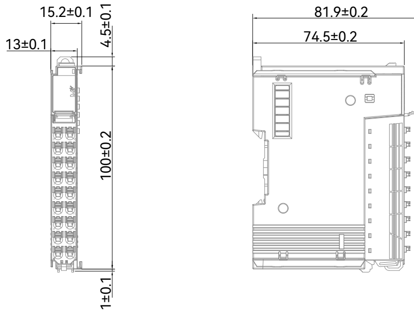
图5 HCMX-ID16-D 模块尺寸图
