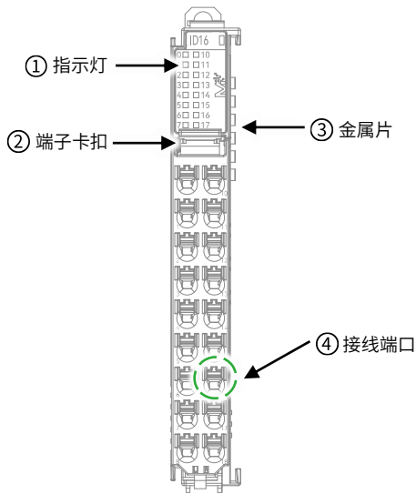
图2 HCMX-ID16-D 正视图部件图
