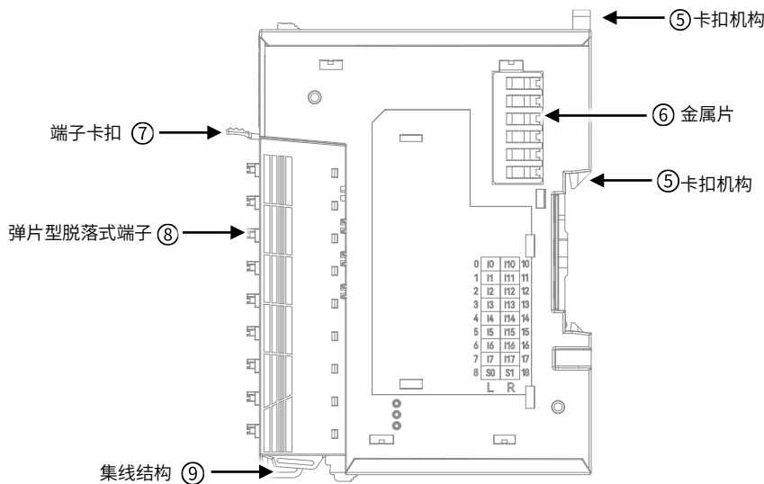
图3 HCMX-ID16-D 模块右视图
