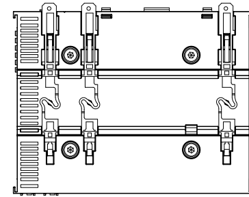
后视图
