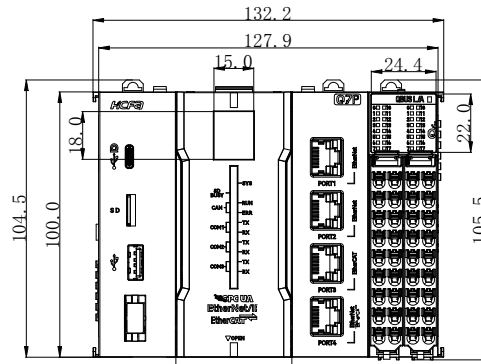
主视图
