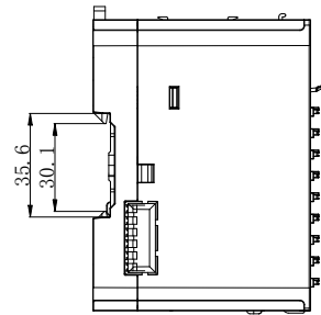
左视图
