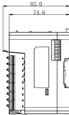
右视图
