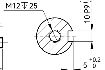
B-B 1:2
