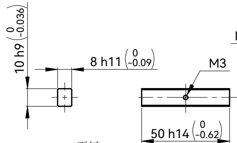
平键 1:2
