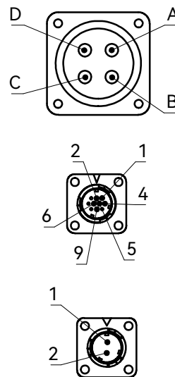
针位 PIN No. 功能定义 Function A U B V C W D C.G
