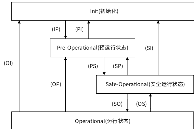
图 4-2, EtherCAT 状态机
