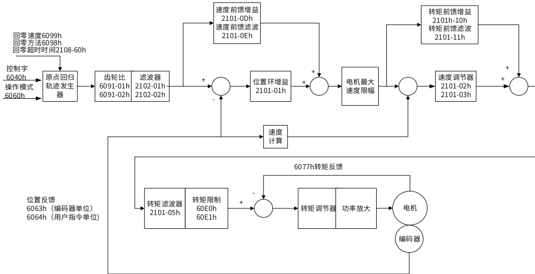
回原模式控制框图
