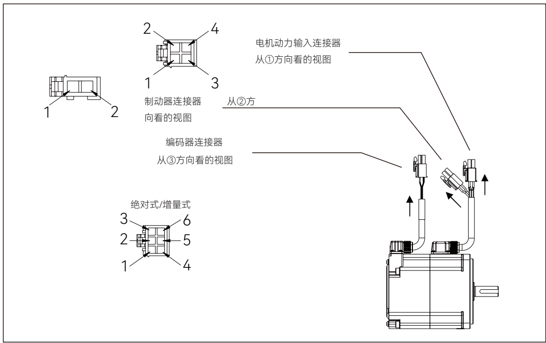
电机连接器和插针排列 (50~750W)
