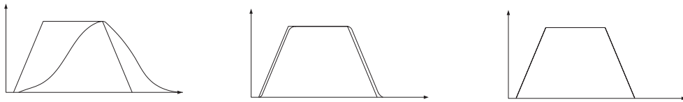
图 6.1 增益定举例
