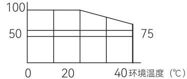
带油封 额定转矩比 (%)
