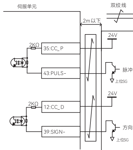
NPN型
