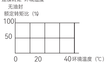
连续转矩-环境温度
