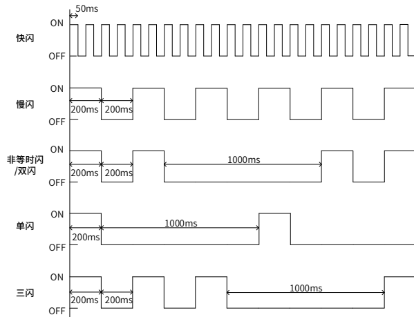
图4 HCQX-EC02-D4 闪烁频率说明图
