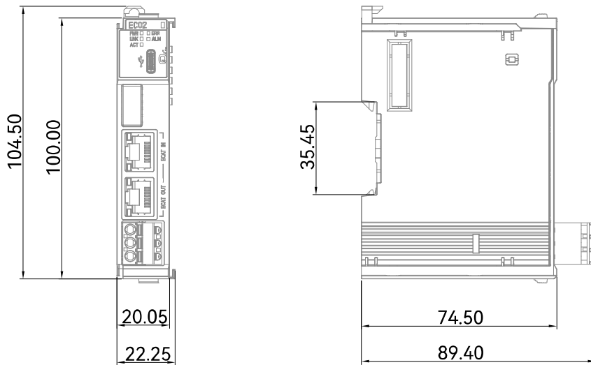
图5 HCQX-EC02-D4 模块安装尺寸 (单位: mm)
