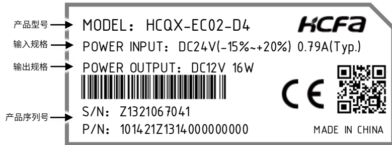
图1 HCQX-EC02-D4型号与标签说明
