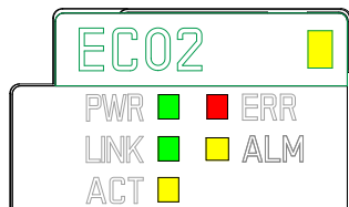
图3 HCQX-EC02-D4 指示灯说明图
