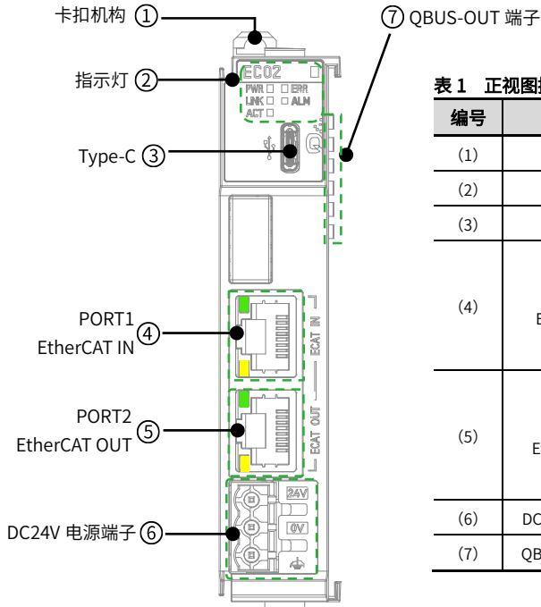
图2 HCQX-EC02-D4 正视图说明图
