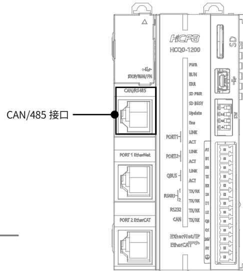
图 5 HCQ0 CPU 单元 CAN/485 接口说明图
