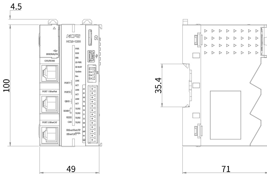
图 8 HCQ0 CPU 模块安装尺寸 (单位: mm)
