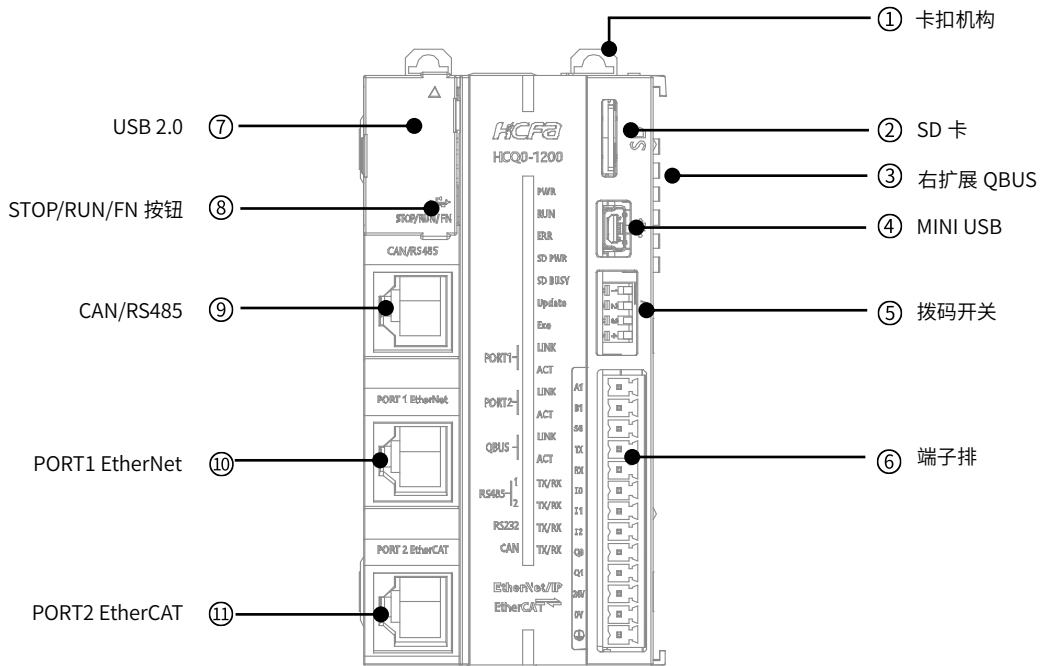
图 2 HCQ0 CPU 单元正视图接口说明图
