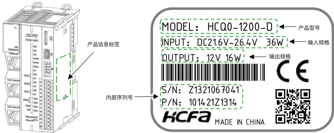
图 1 型号与标签说明
