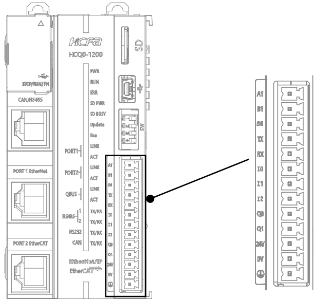
图 3 HCQ0 CPU 单元端子排说明图
