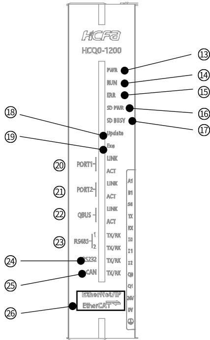
图 7 HCQ0 CPU 单元指示灯说明图
