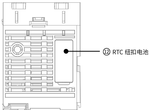
图 6 HCQ0 CPU 单元俯视图接口说明图
