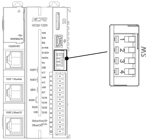
图 4 HCQ0 CPU 单元拨码开关说明图
