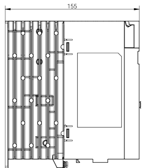
左视图
