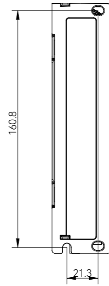
后视图
