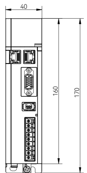
正视图
