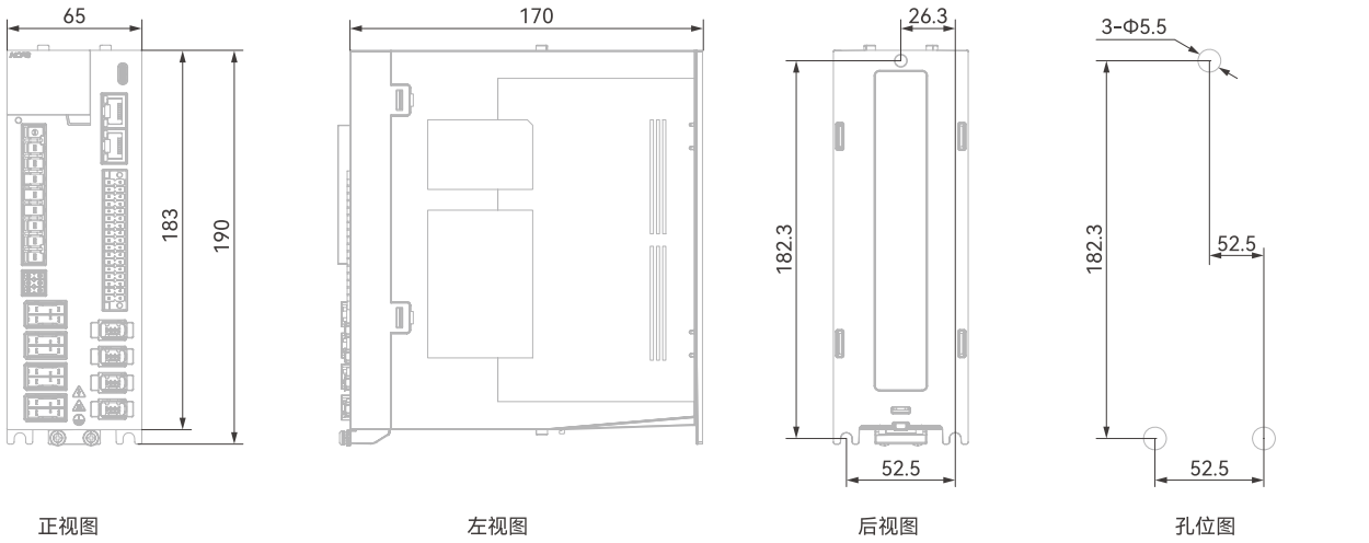
Size B整机外形尺寸（mm）
